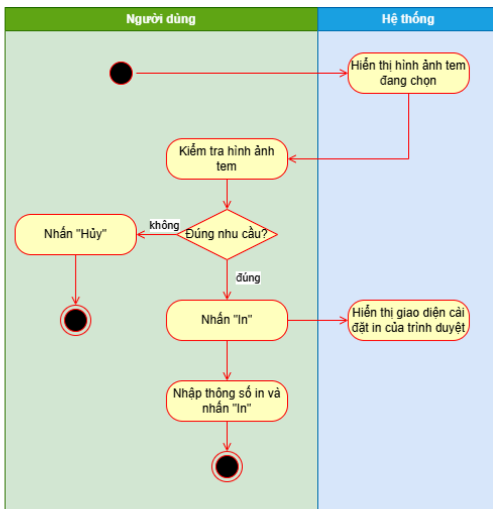
Hình 38 Sơ đồ hoạt động use case In tem lại
