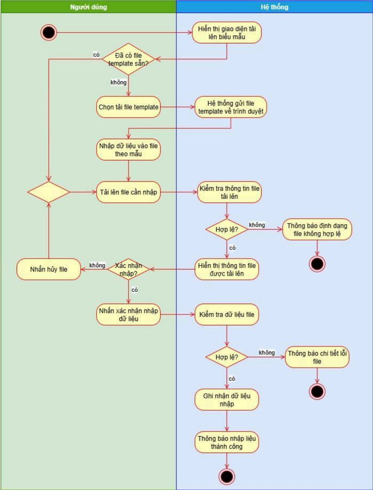
Hình 68 Sơ đồ hoạt động use case Nhập liệu
