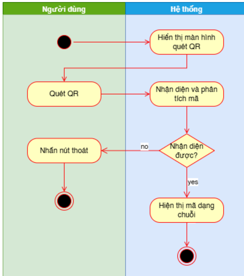
Hình 4 Sơ đồ hoạt động use case Quét QR
