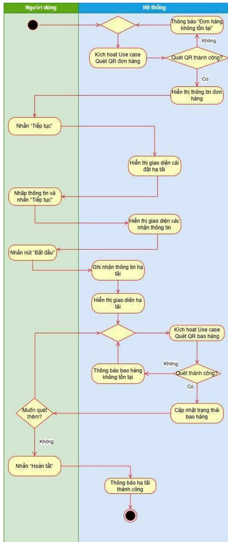
Hình 30 Sơ đồ hoạt động use case Hạ tải
