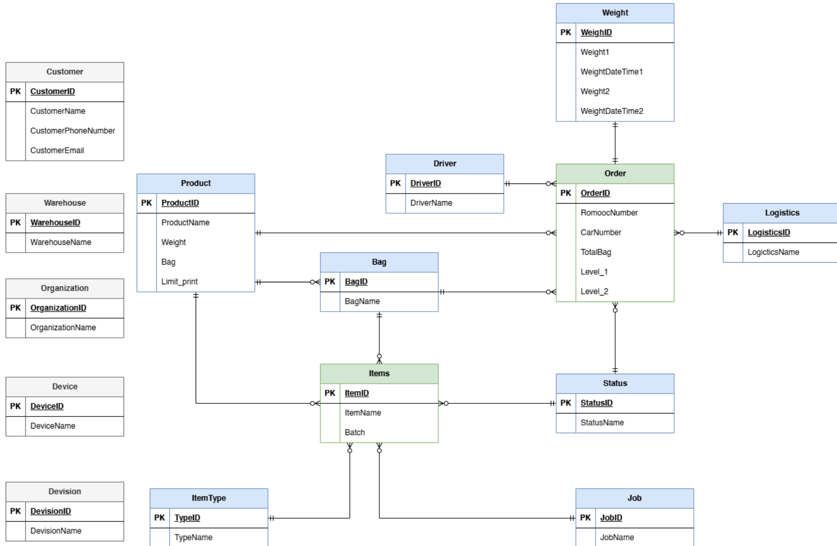
Hình 90 Sơ đồ dữ liệu mức logic
