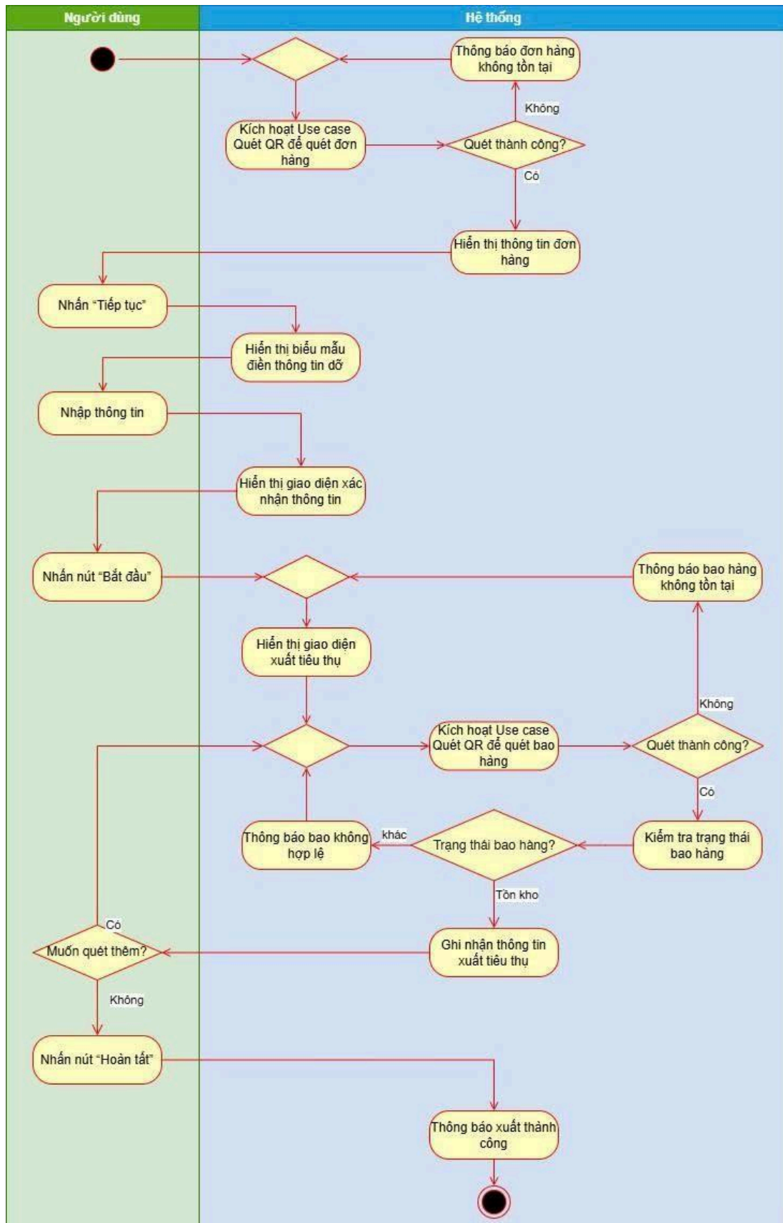
Hình 42 Sơ đồ hoạt động use case Xuất tiêu thụ
