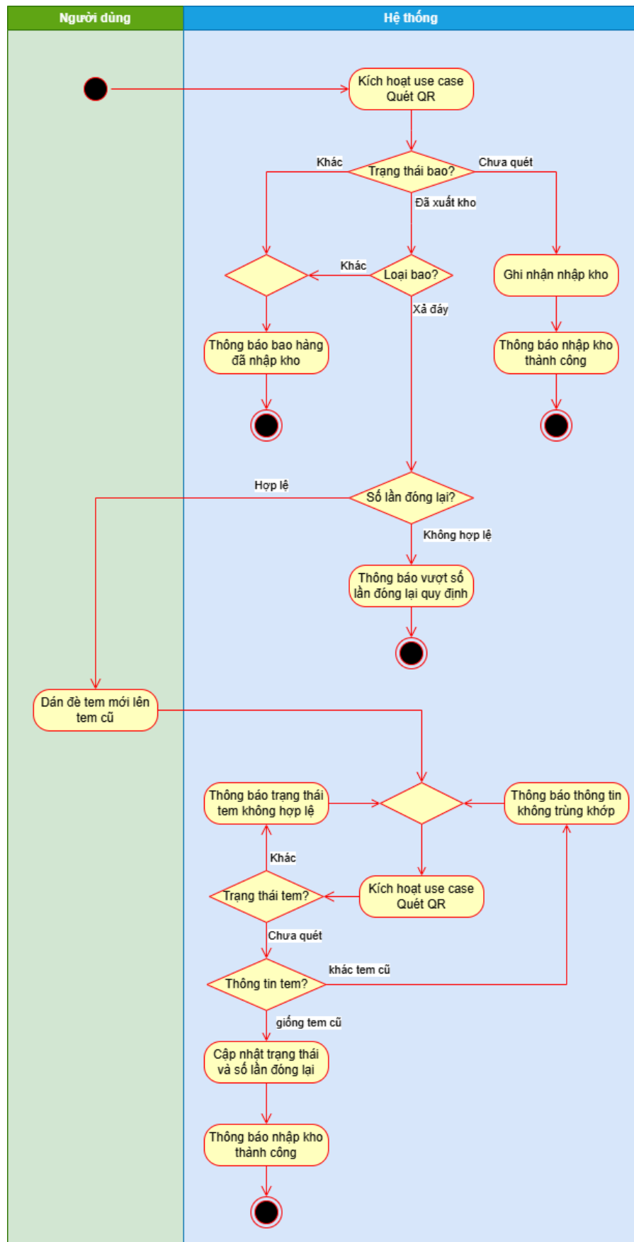
Hình 27 Sơ đồ hoạt động use case Nhập kho
