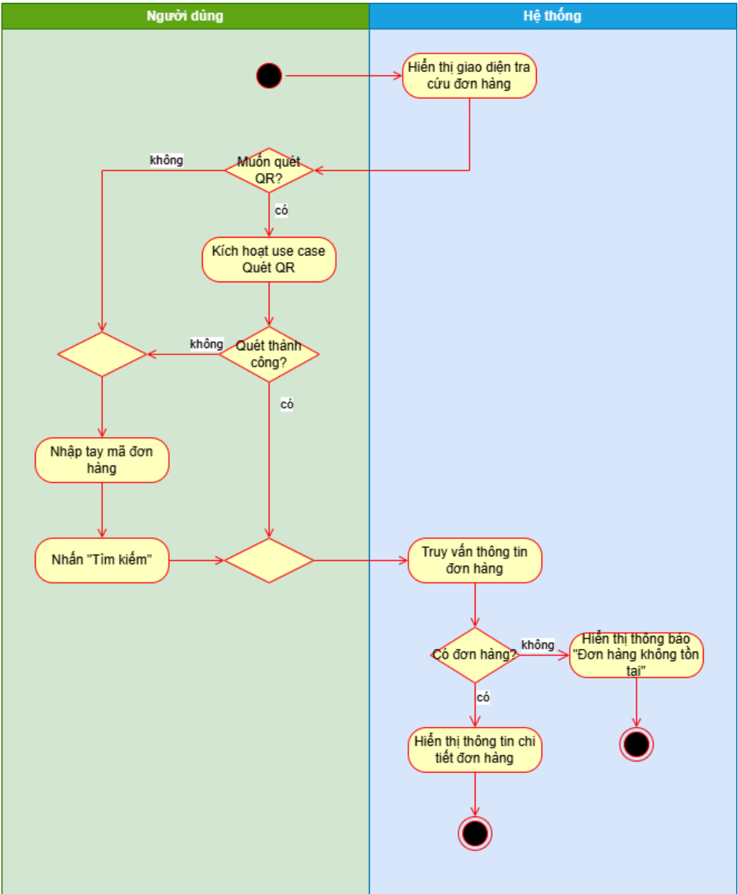
Hình 71 Sơ đồ hoạt động use case Tra cứu đơn hàng
