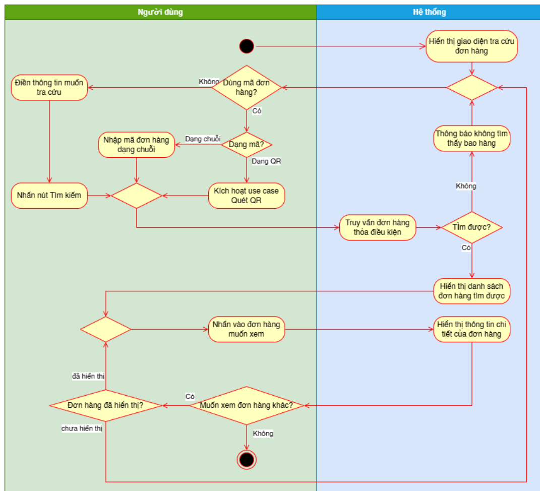
Hình 76 Sơ đồ hoạt động use case Truy xuất đơn hàng
