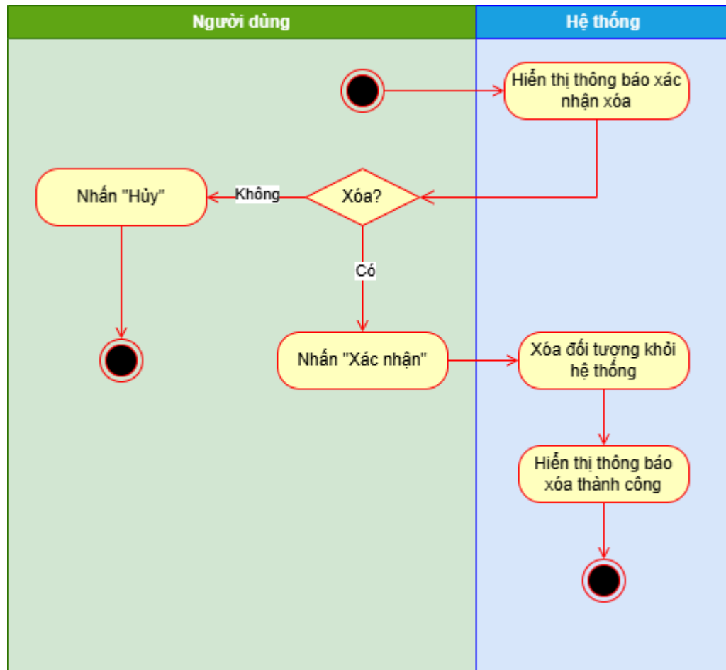
Hình 17 Sơ đồ hoạt động use case Xóa đối tượng
