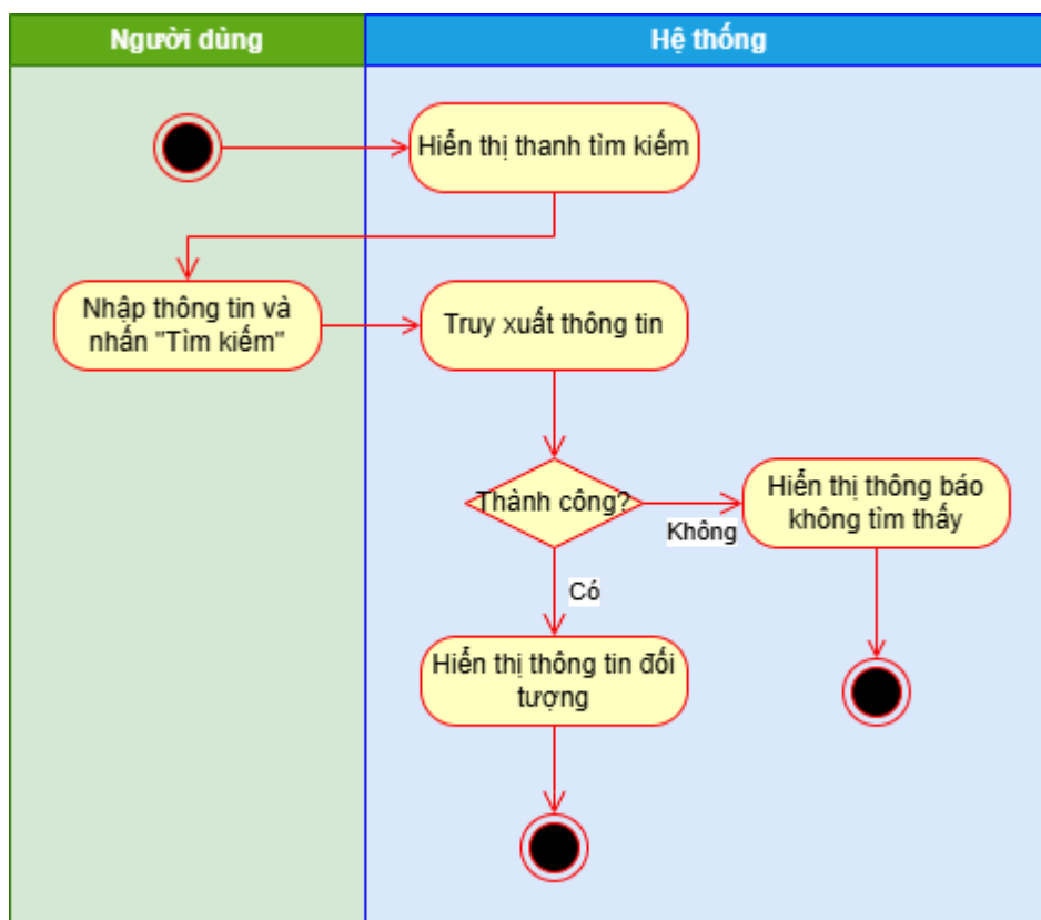
Hình 13 Sơ đồ hoạt động use case Tìm kiếm đối tượng
