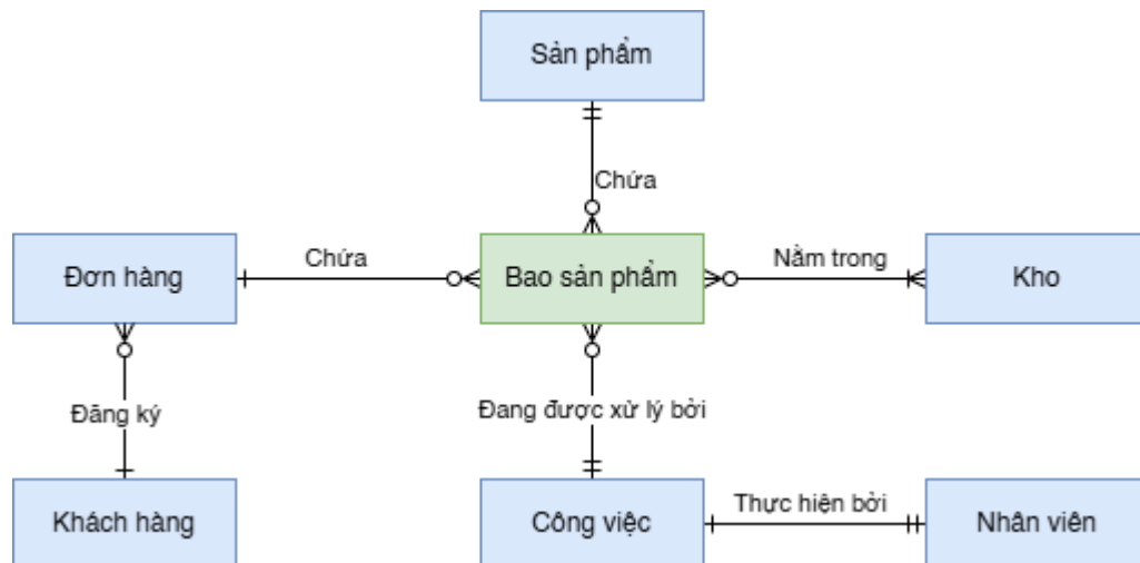
Hình 89 Sơ đồ dữ liệu mức quan niệm
