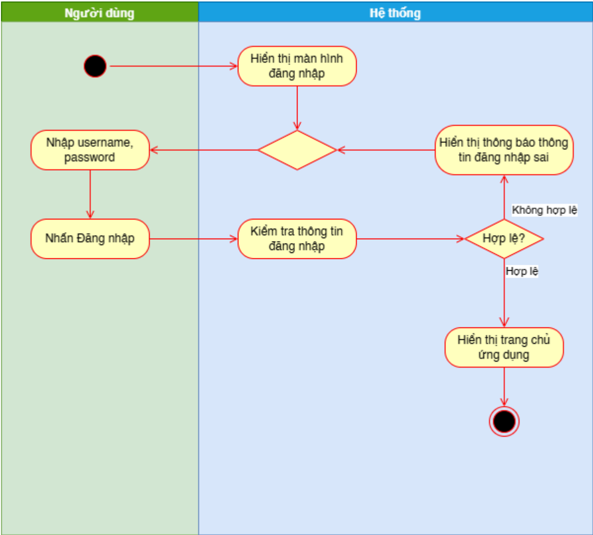
Hình 2 Sơ đồ hoạt động use case Đăng Nhập
