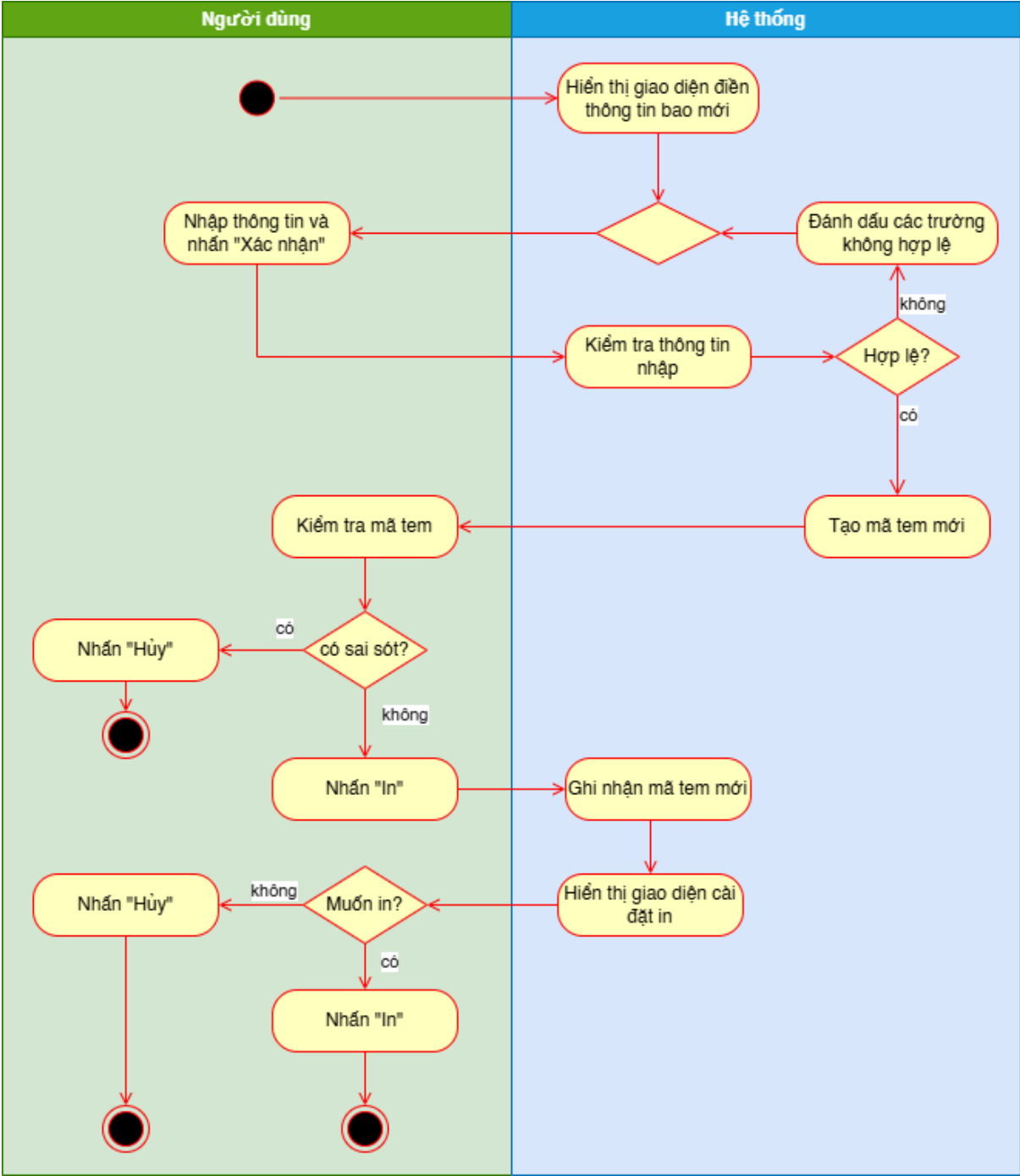
Hình 36 Sơ đồ hoạt động use case Tạo tem mới
