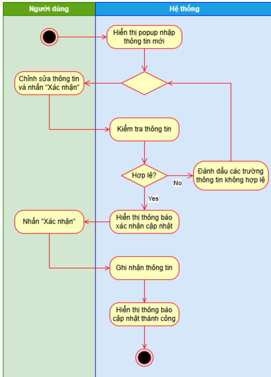
Hình 20 Sơ đồ hoạt động use case Sửa đối tượng
