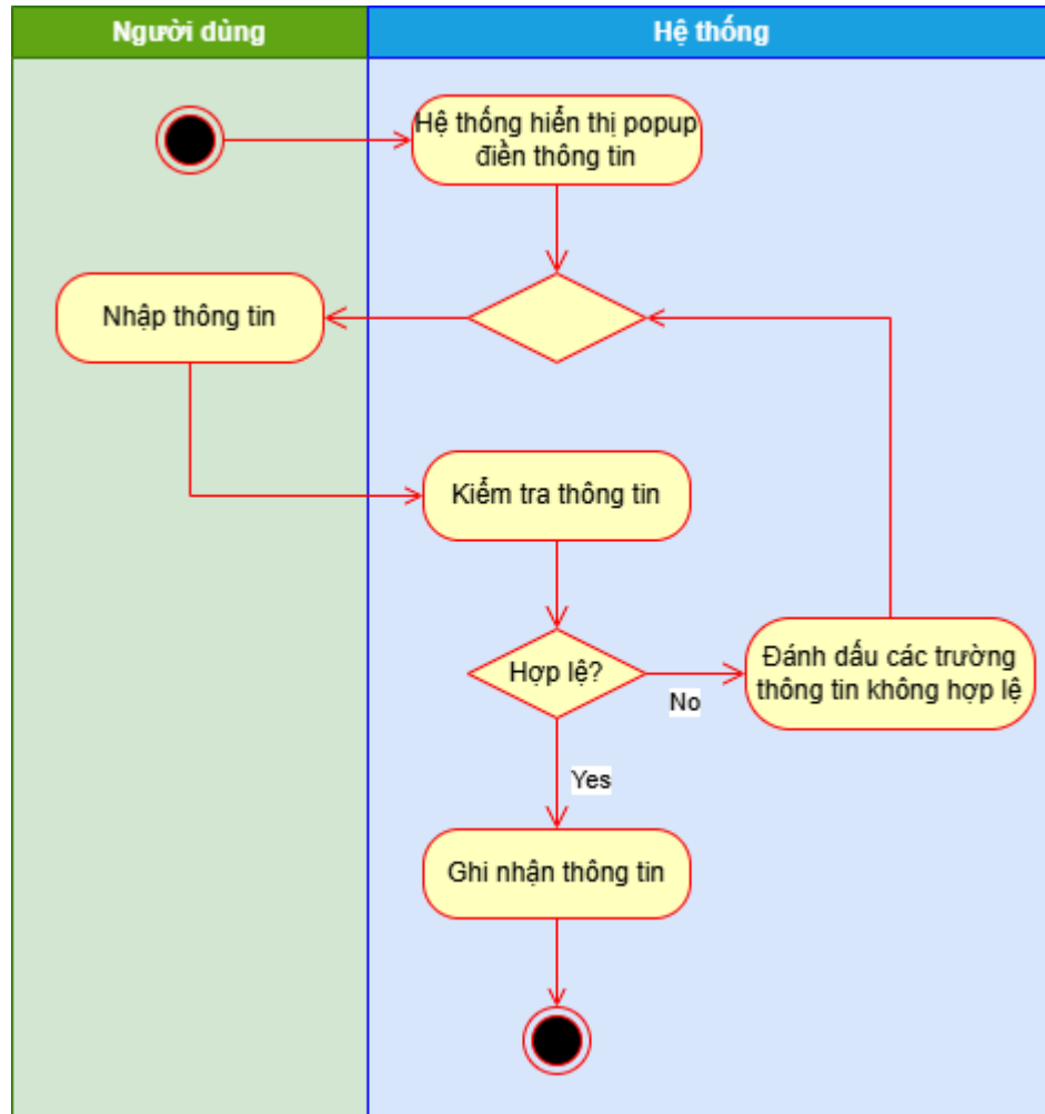
Hình 15 Sơ đồ hoạt động use case Thêm đối tượng
